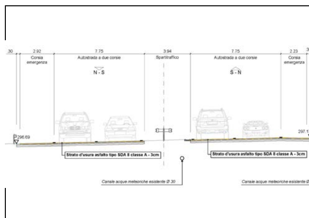
Sezione tipo
