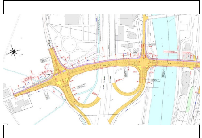
Anschluss A14 Gisikon-Root, Situation
